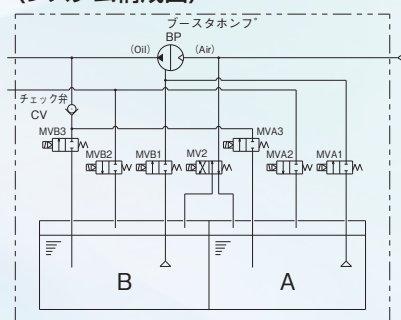
〈システム構成図〉
